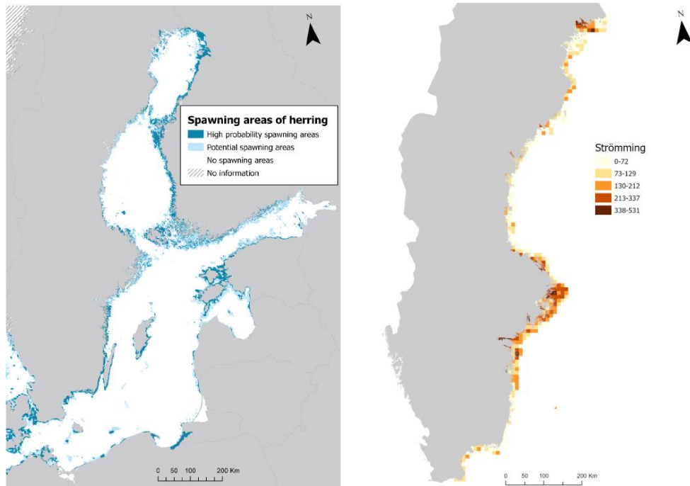
Figur 4. Till vänster: potentiella lekområden för strömming i Östersjön utgående från översiktlig karta över vegetationsklädda bottnar (figuren är från Bergström m.fl. 2021). Till höger: modellerade uppväxtområden för strömming längs svenska kusten från Hanöbukten till Norrbotten baserade på högupplöst information på fiskförekomst och habitatvariabler. För tydligare visualisering har modellprediktionerna i den högra kartan aggregerats till en cellstorlek om 5x5 km (figuren från Erlandsson m.fl. 2021). Lek- och uppväxtområden förekommer längs hela ostkusten, där de stora skärgårdarna utgör de viktigaste områdena.
